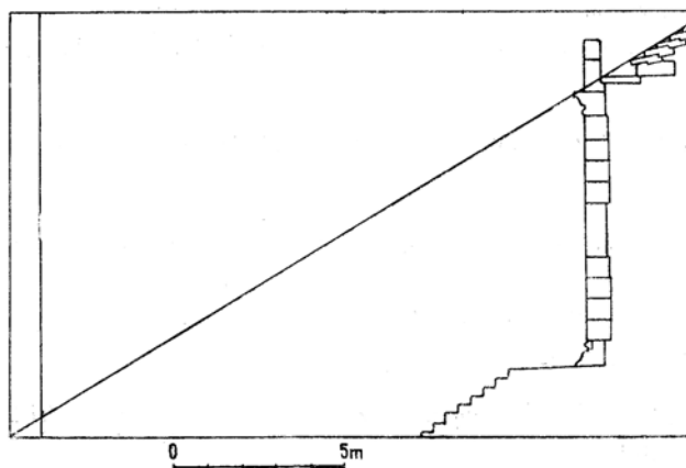
Fig. 2 – Secțiune a paramentului cu așezarea mediană, în construcție(?) a asizei metopelor; ( apud SÂMPETRU 1984, p. 69).
