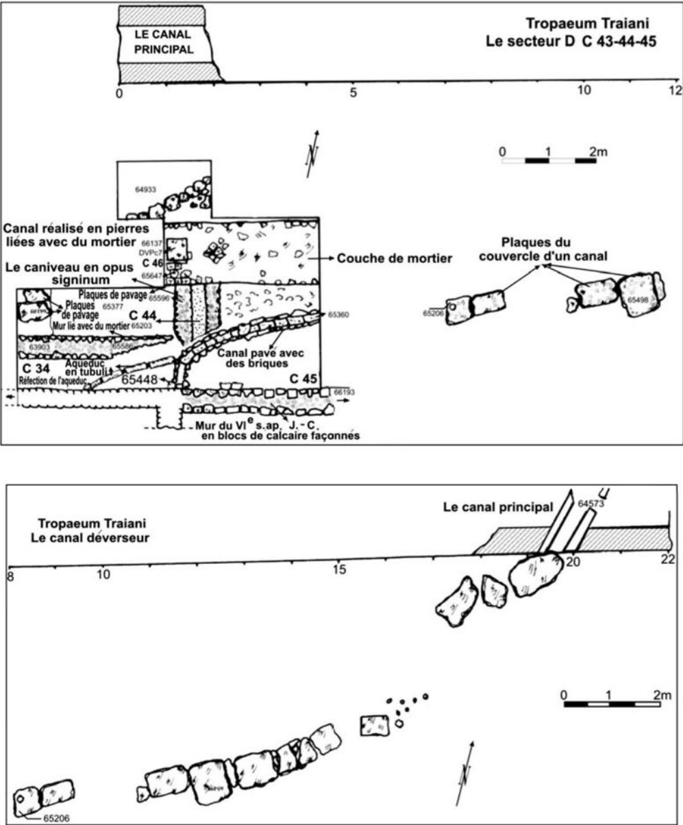
Fig. 6 - Plan de situation: les systèmes d'adduction et d'évacuation de l'eau, Via Principalis , Secteur D, 2005.
