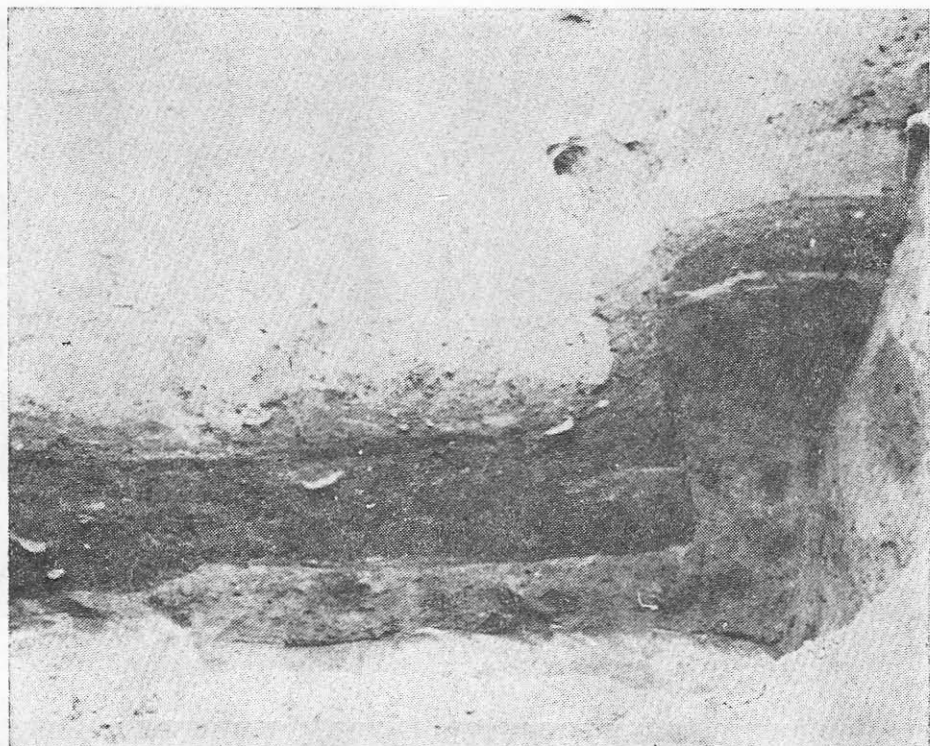
Fig. 23. Profilul locuinței-bordei nr. 2 din O-sud.
