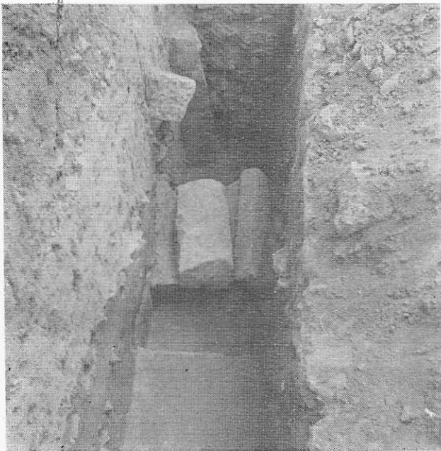
Fig. 4. Secțiune de-a lungul axului bazilicii „simple” (A) : 1-2, pavaj și zid (sec. IV e.n.) ; 3, piese arhitectonice (sec. II-III e.n.) ; 4, baza pentru balustrada cancelli altarului.
