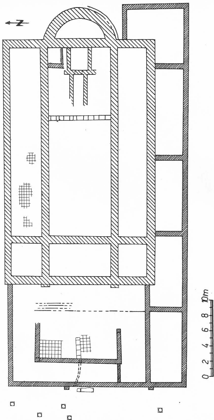
Fig. 1. Tropaeum Traiani : bazilica „simplă” (A) : plan.
