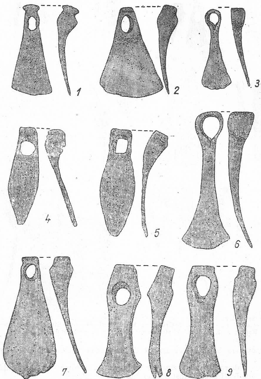
Fig. 2. Sape și săpăliși dacice (sec. I î.e.n.—sec. I e.n.), 1, 4—7 Grădiștea Muncelului; 2, Lunca-Deva; 3 Tilișca-Sibiu; 8, 9 Piatra Craivii (lângă Alba-Iulia).
