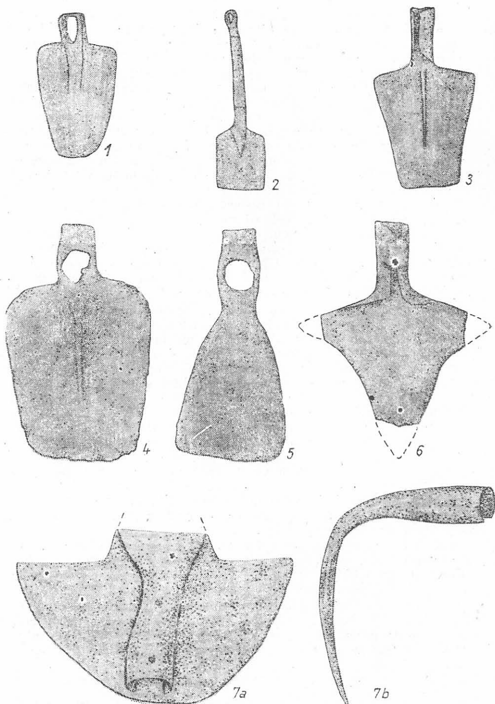
Fig. 5. Sape, săpăliși (1, 4, 5, 7) și hirlțe-lopeți (2, 3, 6) din epoca romană. 1 Sucidava-Celei; 2. Pandantiv al colierului de aur din tezaurul nr. 1 de la Șimleul Silvaniei (sec. III—IV e.n.); 3 Moșneni-Peceneaga, lângă Mangalia (sec. I—II e.n.) 4, 5, 7 Gornea, jud. Caras-Severin (sec. IV e.n.); 6 Răcari jud. Dolj (sec. II—III e.n.)
