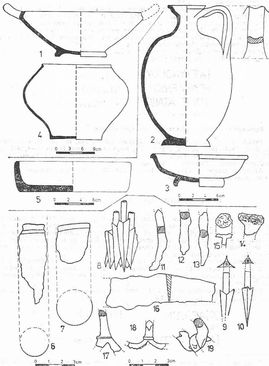
Fig. 2: 1-3 — lékane, lekythos și bol de la Medgidia; 4-5 — urnă și capac de la Făurei; 6-19 — obiecte de fier din mormintul de la Mangalia (6-7 fragmente din tubul de înmănușare al unui virf de lance); 8-10 — virfuri de săgeată; 11-14 — pi-roane; 15 — țință; 16 — lamă de cuțit; 19 — zale de lanț (?).
