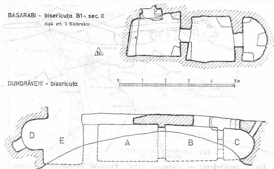
Fig. 3. Planurile bisericuțelor B 1 de la Basarabi-Murfatlar și de la Dumbrăveni.
