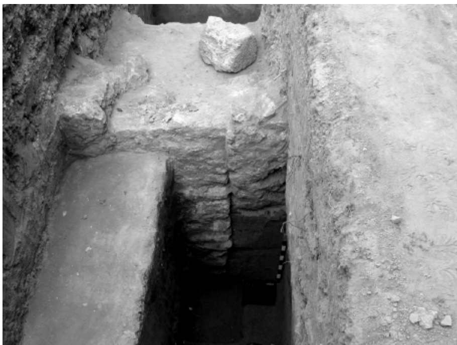
Fig. 5 - a. Fundația zidului de incintă surprinsă în SI. Vedere dinspre sud
