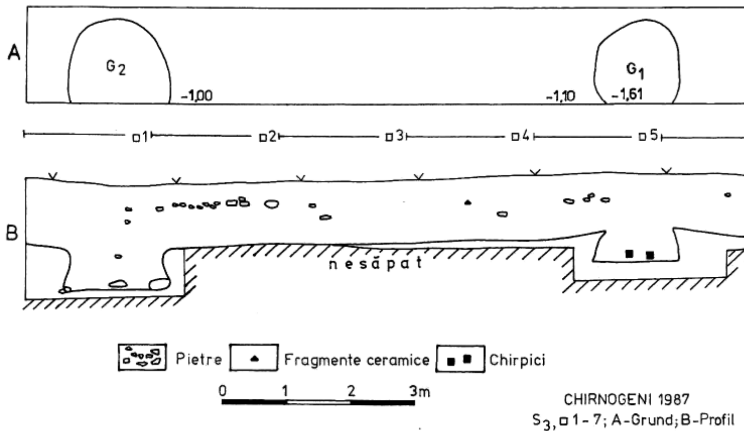
Pl. IV - Plan și profil al secțiunii S III, c. 1-6 (parțial) cu gropile G 1 și 2.
